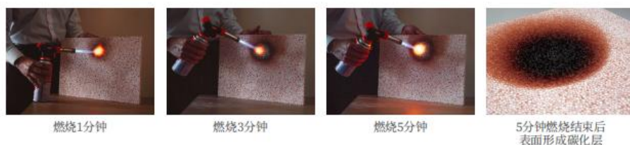
真金板裸板1300℃喷灯燃烧试验
